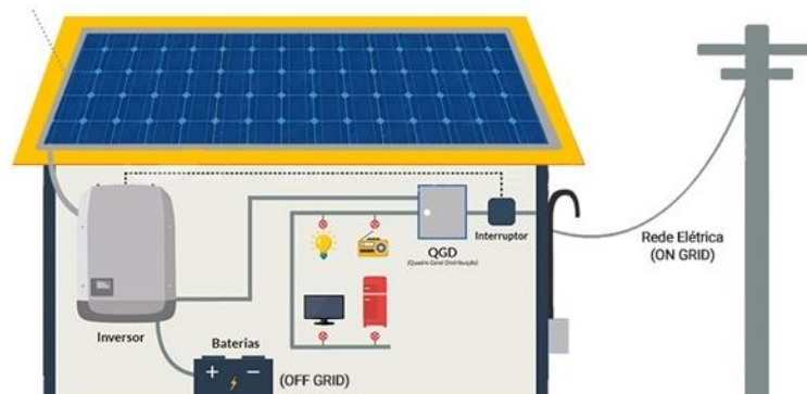
Figura 20 – Diagrama de instalação e funcionamento de sistemas híbridos
