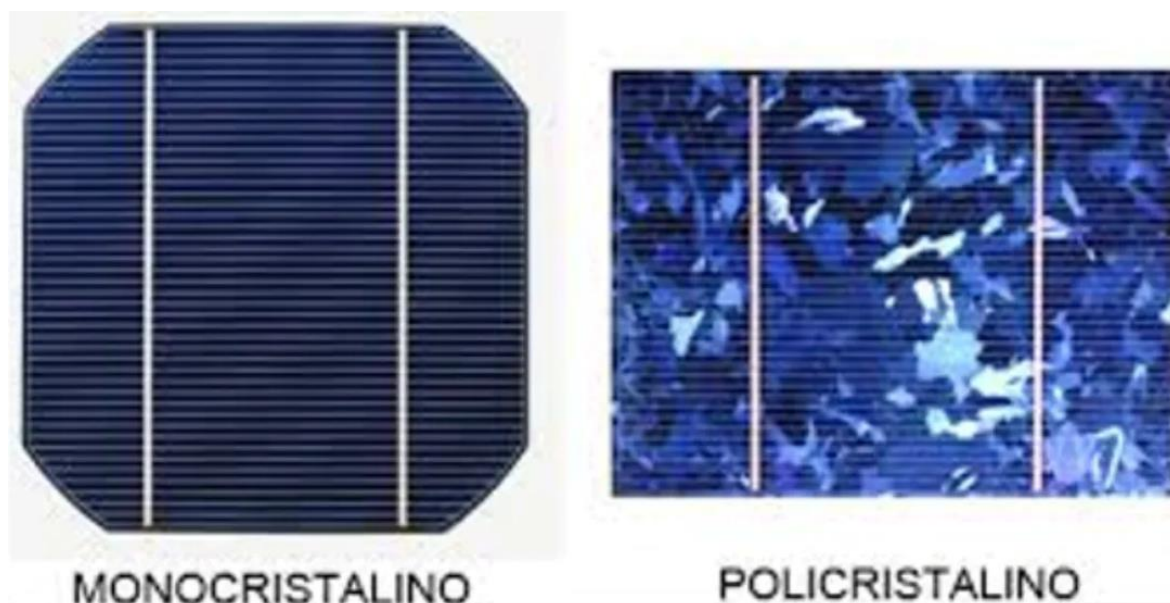
Figura 6 – Diferença entre monocristalino e policristalino
